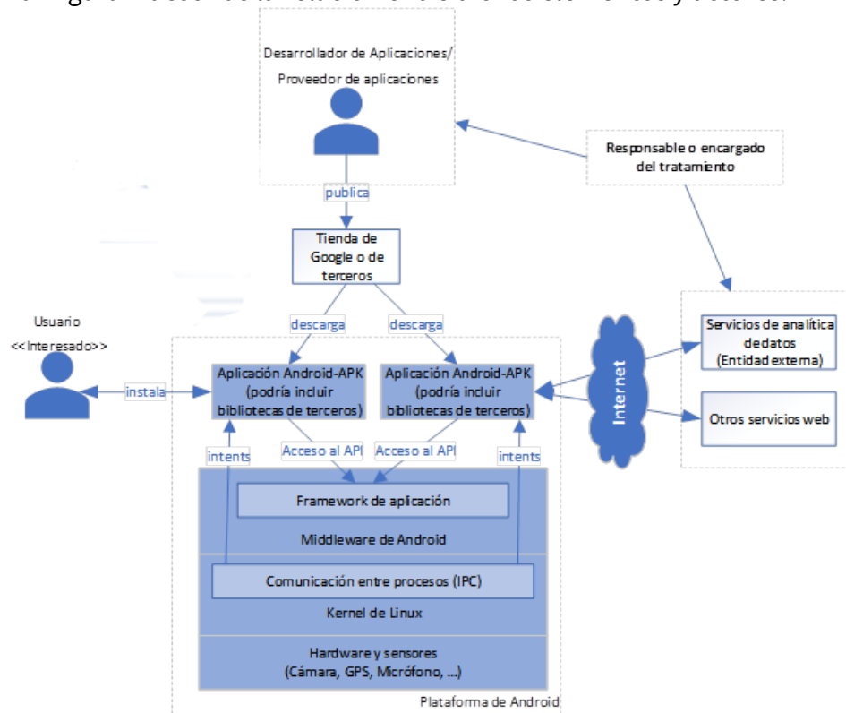
Figura 1. Ecosistema Android
